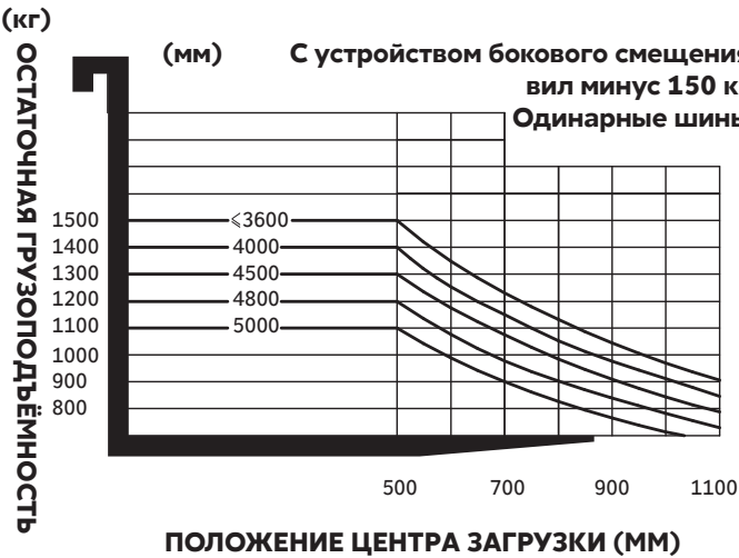
График падения грузоподъёмности CPD18FVL CPD20FVL
